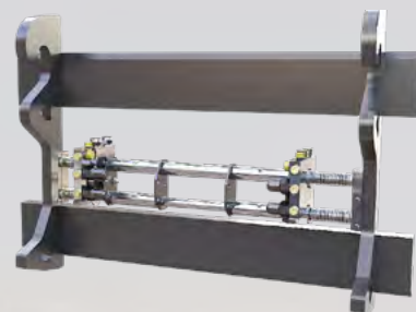
ADAPTATEUR ISO
